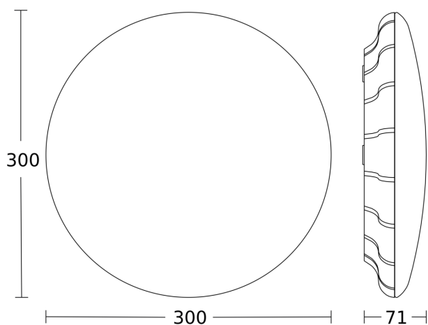
Dessin dimensionnel 1
